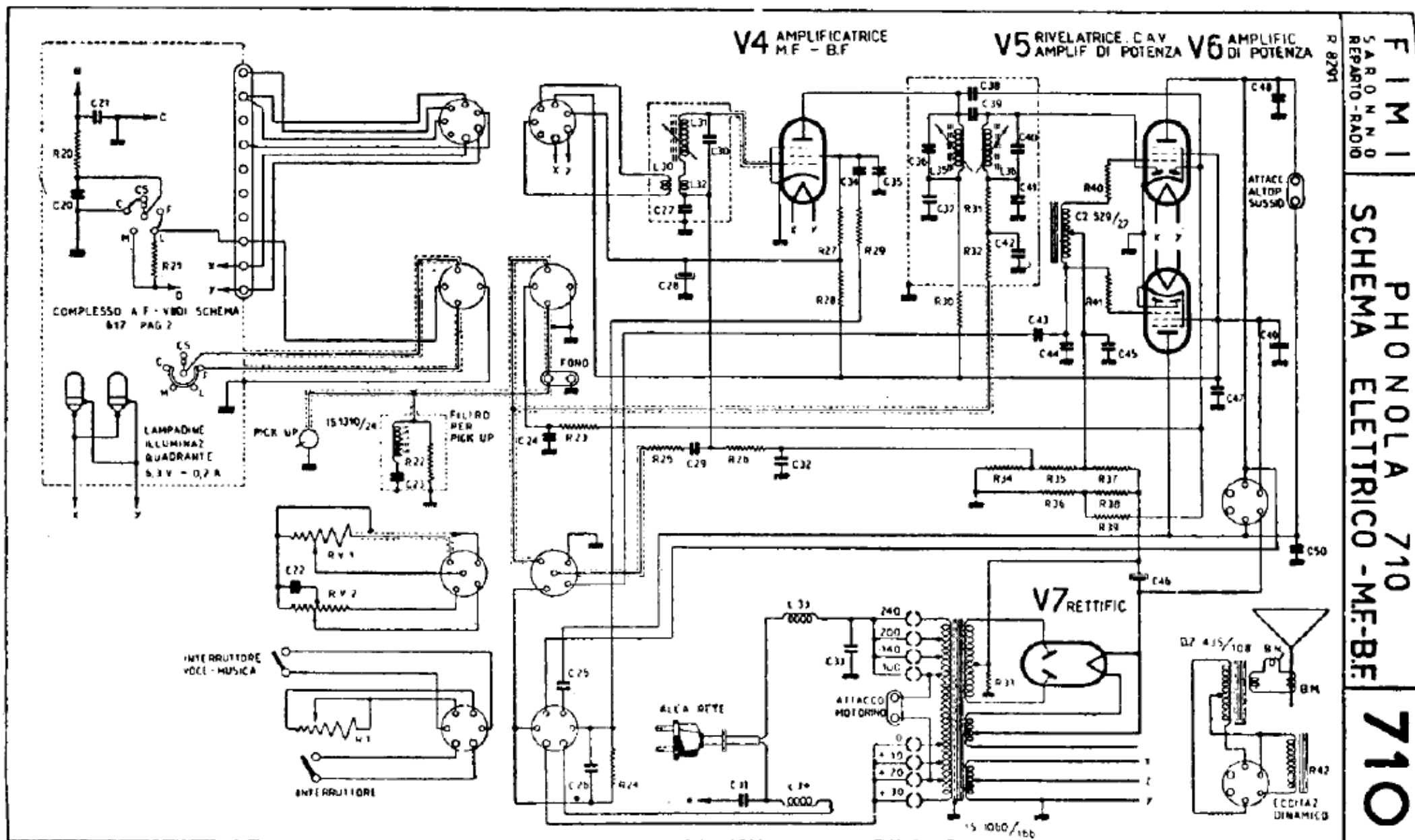
PHONOLA (S. A. FIMI). — Mod. 710. — Compl. MF e BF. (Compleso A. F. quello del mod. 617). — Produzione 1939. Media frequenza: 470 kHz.
